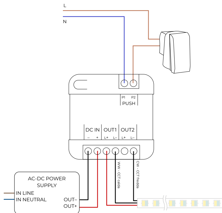
FIG. 15 - collegamento pulsante a tensione di rete
