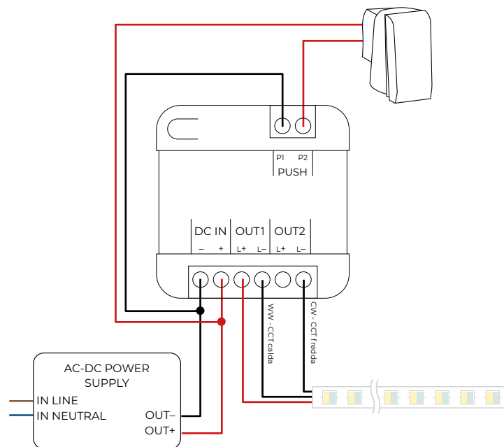
FIG. 16 - collegamento pulsante con tensione proveniente dall'alimentatore
