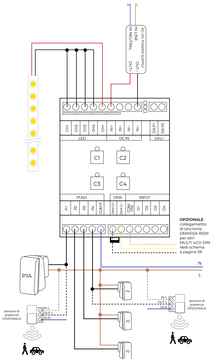
FIG. 28 - collegamento Temporizzato/Garage Mode 1 uscita
