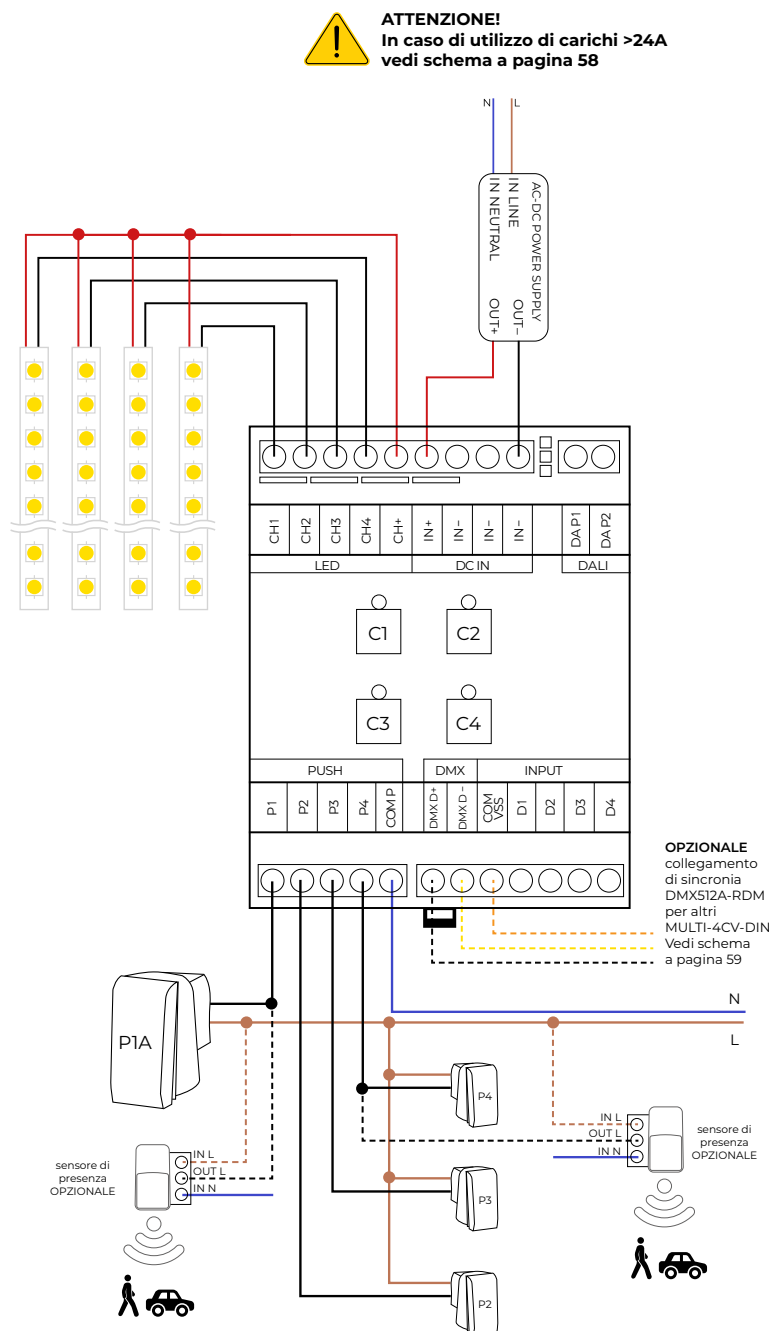
FIG. 29 - collegamento Temporizzato/Garage Mode 4 uscite
