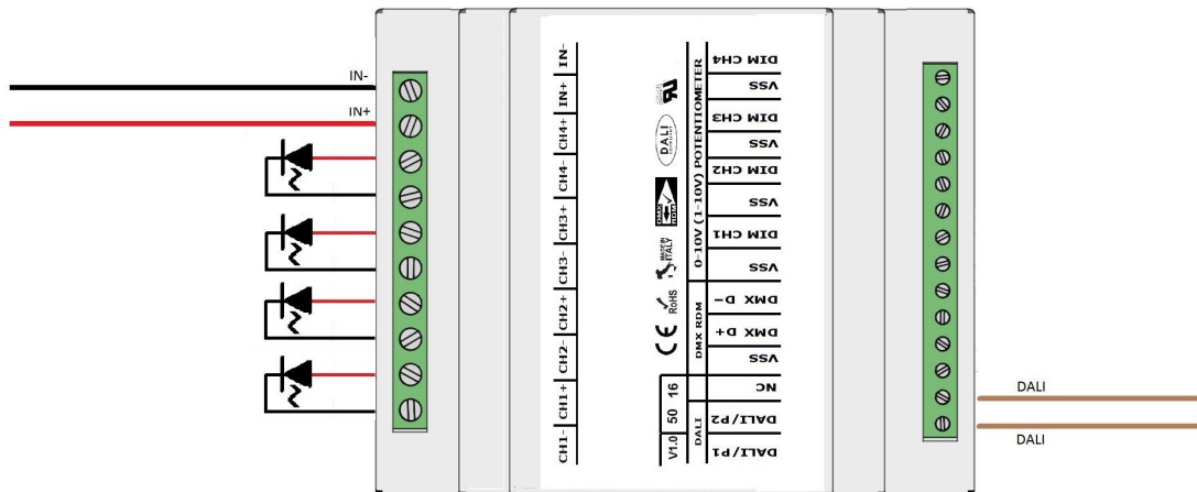
COLLEGAMENTO DALI L405MA02C4A01 - FIGURA N. 7
