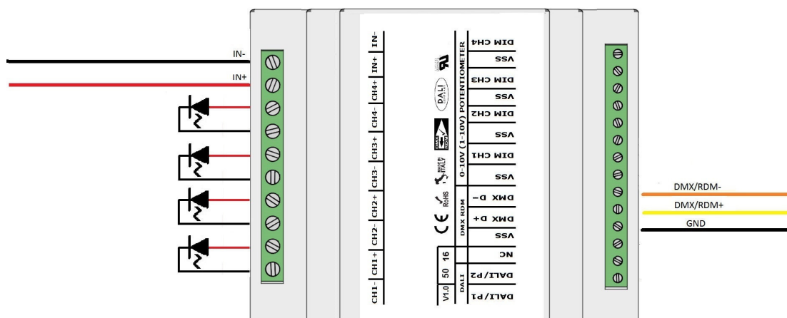
COLLEGAMENTO L405MA02C4A01 A BUS DMX512/RDM - FIGURA N. 3
