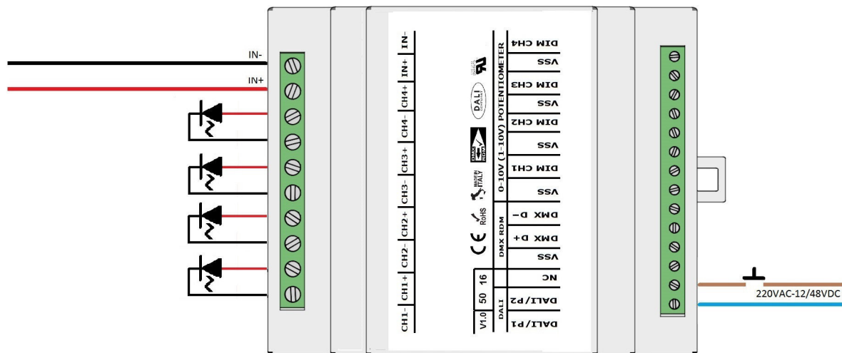
COLLEGAMENTO PULSANTI L405MA02C4A01 - FIGURA N. 9
