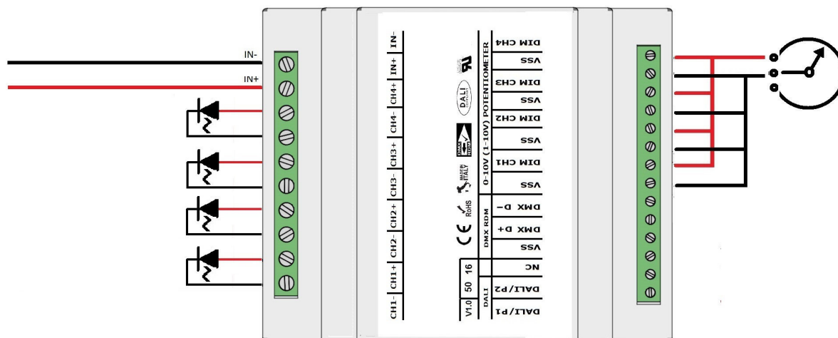
COLLEGAMENTO POTENZIOMETRO MONOCANALE L405MA02C4A01 - FIGURA N. 12
