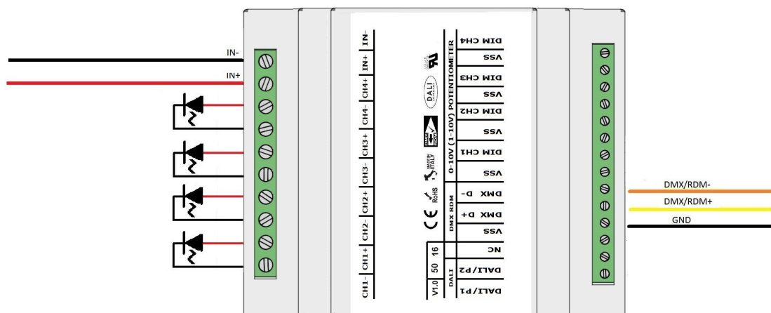
COLLEGAMENTO L405MA02C4A01 A BUS DMX512/RDM - FIGURA N. 5
