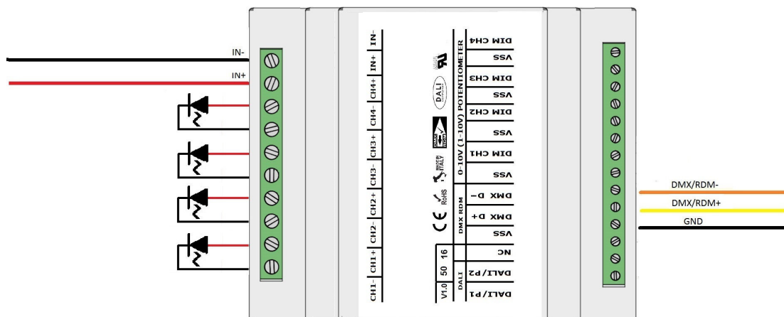
COLLEGAMENTO L405MA02C4A01 A BUS DMX512/RDM - FIGURA N. 2
